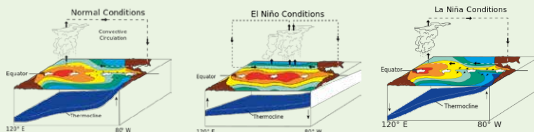
Figure 2.1 The El Niño Southern Oscillation (ENSO) phenomenon.
